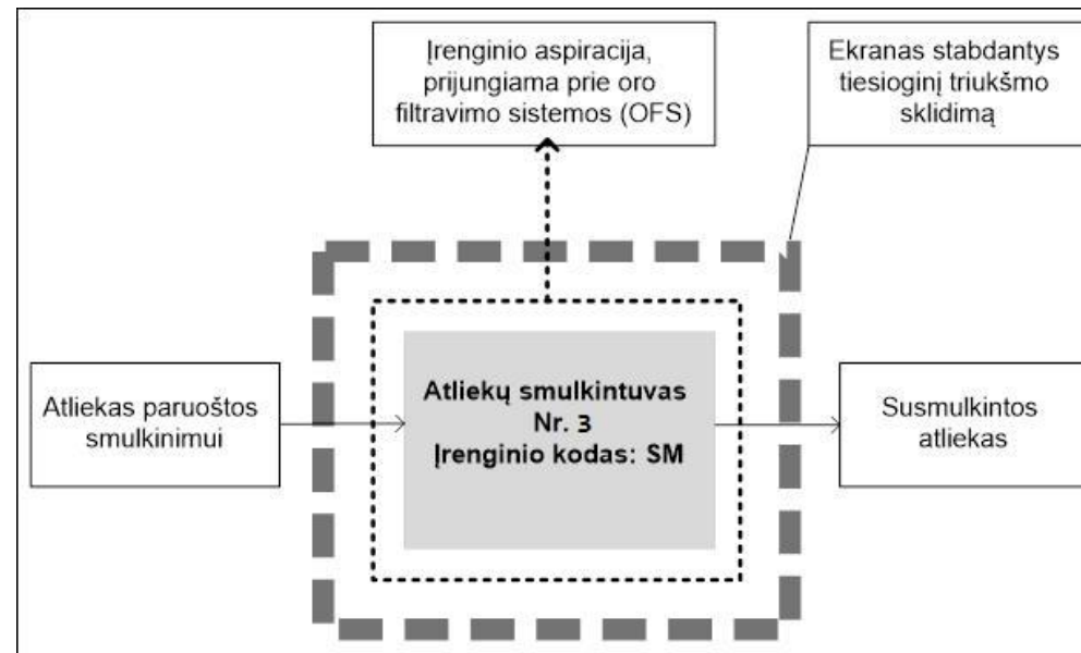
2-8 pav. Atliekų smulkintuvas Nr. 3
